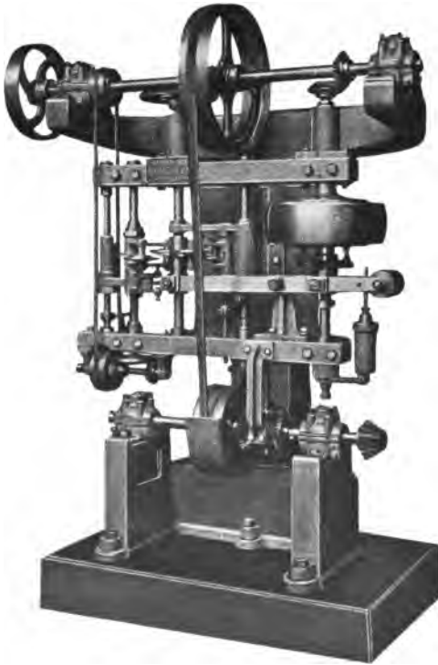
Fig. 62. Turbinenregulator.
